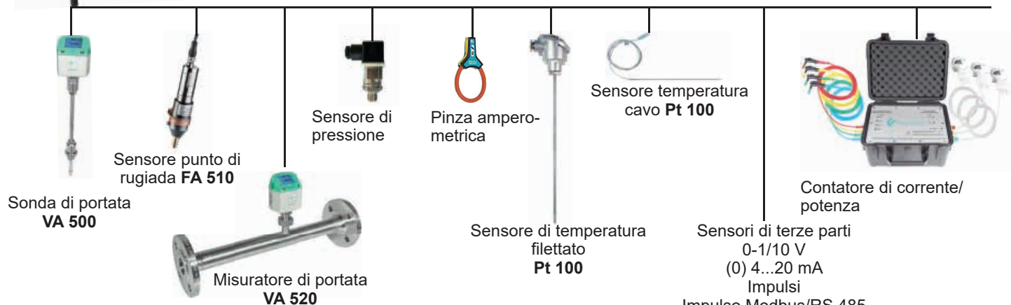
Secondo ingresso sensore a scelta per sensori esterni (solo DP 510)
